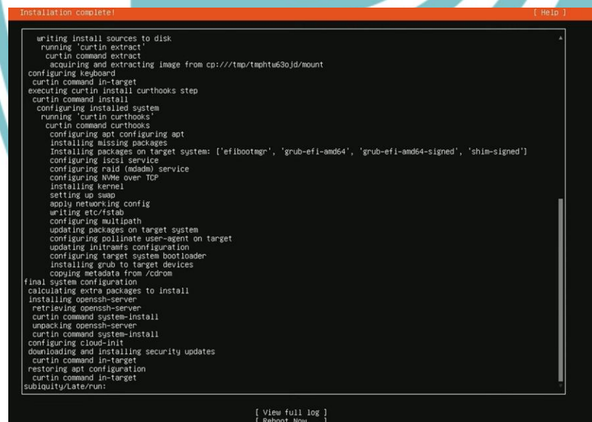
Gambar 4.17 Instalasi Akhir Ubuntu
